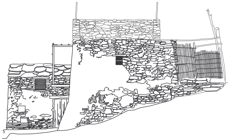
PROSPETTO SUD
